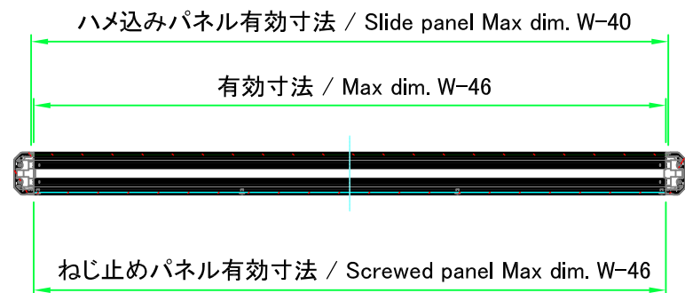
A-A (1:8)
